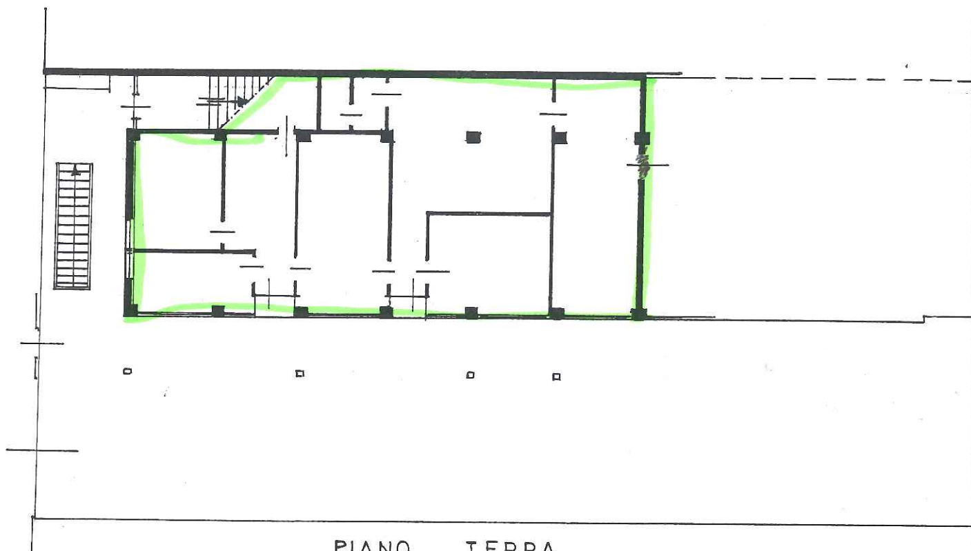
PIANO TERRA H. 3.10
